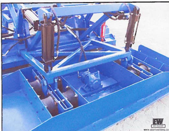
Photo 2.14 Plaques vibrantes arrière de type courant
