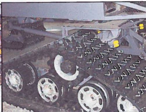
Photo 2.27 Exemple de chenille en caoutchouc
