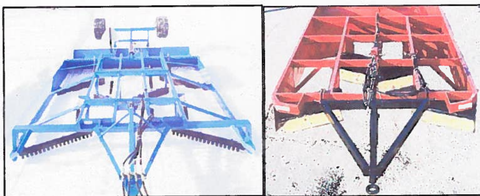
Photo 2.3 Châssis à lames multiples de type courant et modèle de lames
