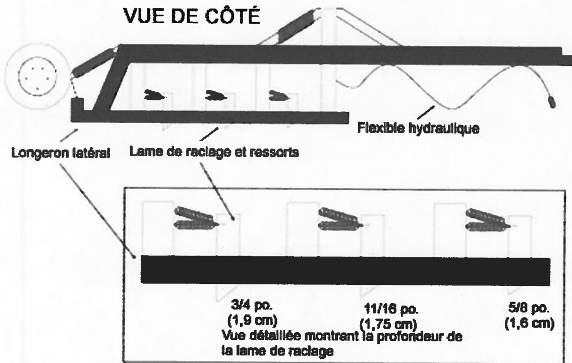
Figure 2.2 Conception de traîneau niveleur à lames multiples de type courant — vue de côté avec vue agrandie des lames de raclage
