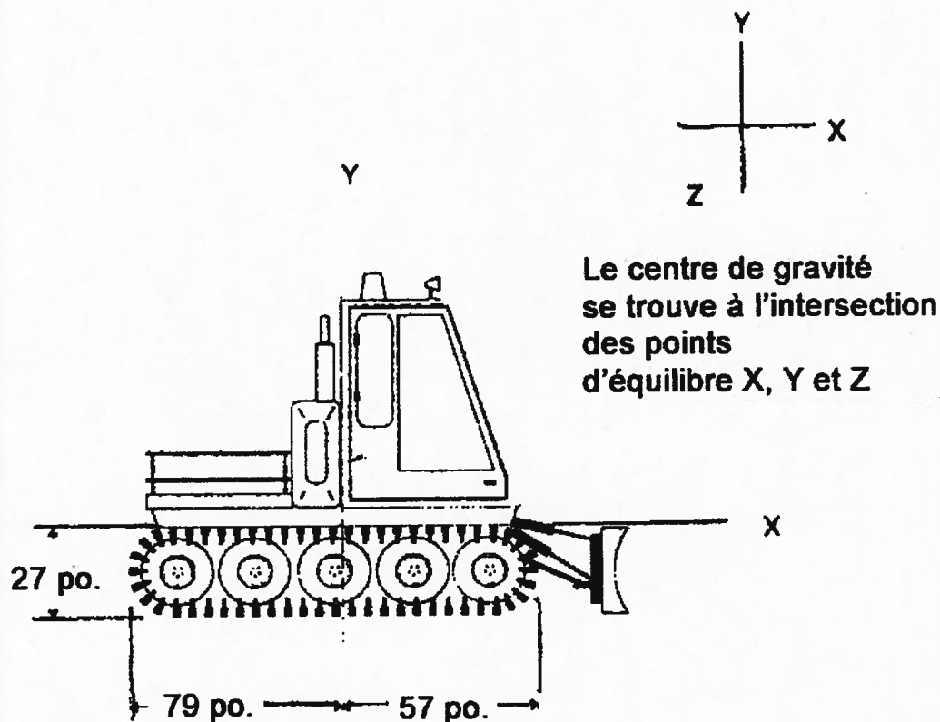
Figure 2.4 Centre de gravité d'un tracteur de damage à deux chenilles, de type courant
