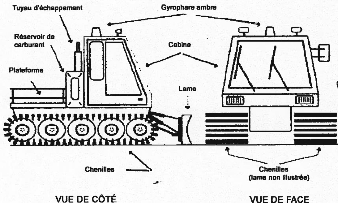
Figure 2.3 Composants classiques d'un tracteur de damage
