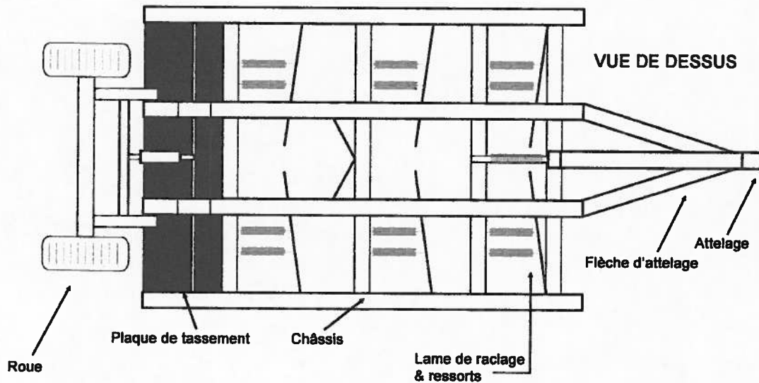
Figure 2.1 Conception de traîneau niveleur à lames multiples de type courant — vue de dessus
